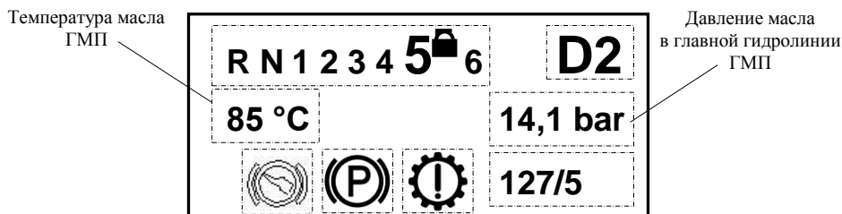
Рисунок 4 – Основной экран №3
