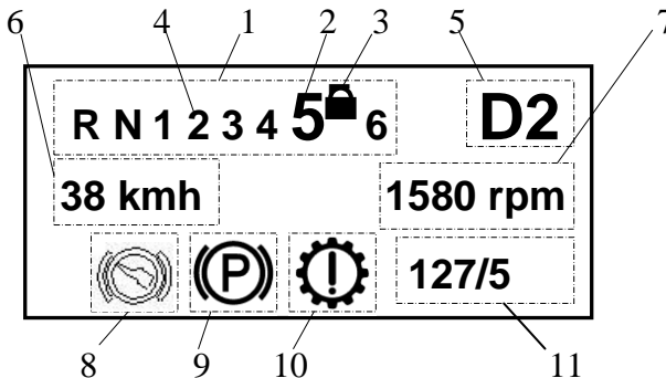
Рисунок 2 – Основной экран №1: 1 – индикаторы передач ГМП; 2 – передача, включенная в текущий момент времени (крупный шрифт); 3 – индикатор блокировки ГТ; 4 – передачи, на которых разрешено движение (мелкий шрифт); 5 – индикаторы режима, заданного селектором передач; 6 – скорость автомобиля; 7 – частота вращения двигателя; 8 – индикатор рабочего тормоза; 9 – индикатор стояночного тормоза; 10 – индикатор неисправности в ГМП; 11 – код обнаруженной неисправности
